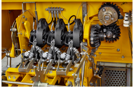
3 ipli Alman Rasspe marka bağlama düzeneği
