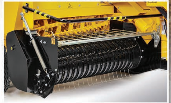
BC 5040 ve BC 5040 HB modellerinde hidrolik olarak kontrol edilen 155 cm toplama genişliği ile etkin toplama performansı
