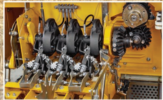
3 ipli Alman Rasspe marka bağlama düzeneği
